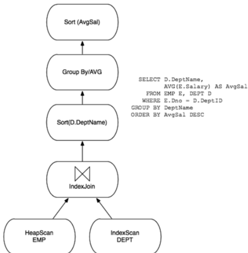
图 4-1 一个查询计划
