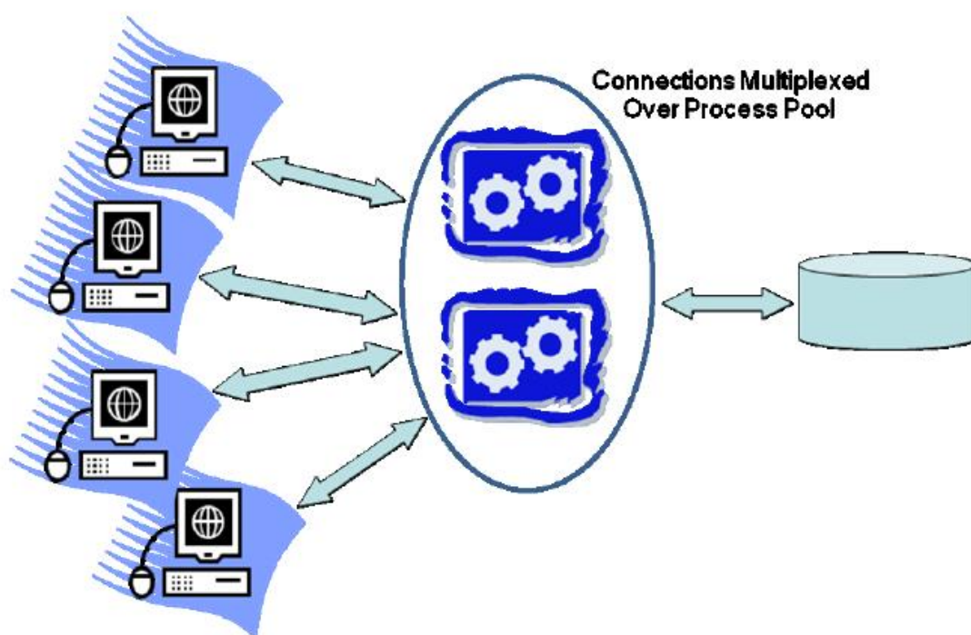
图 2-3 进程池
